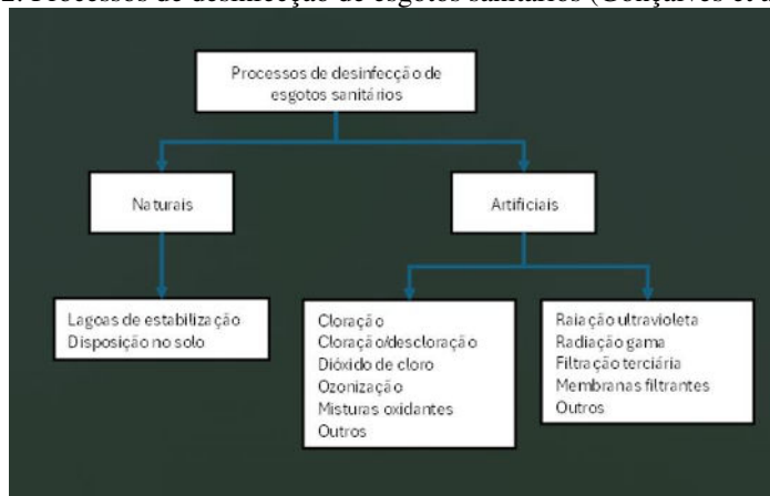
Figura 2: Processos de desinfecção de esgotos sanitários (Gonçalves et al, 2003).
