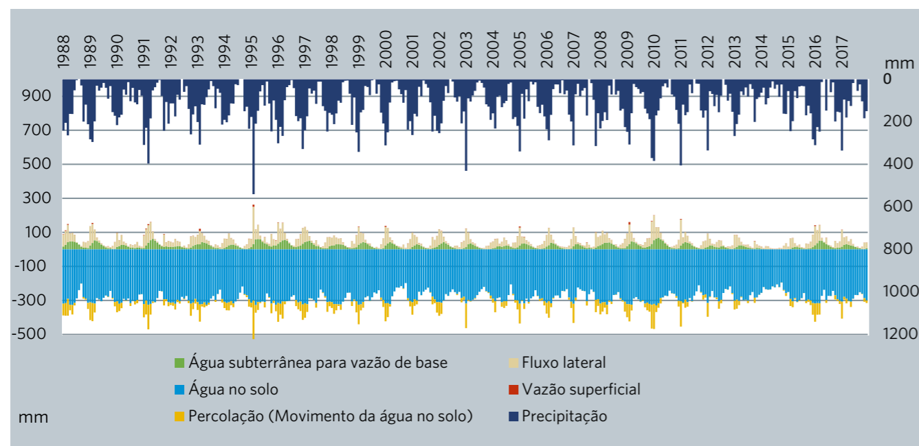
FIGURA 10: COMPONENTES DO BALANÇO HÍDRICO NOS RESULTADOS DO MODELO SWAT PARA A LINHA DE BASE NA SUB-BACIA DO JAGUARI
