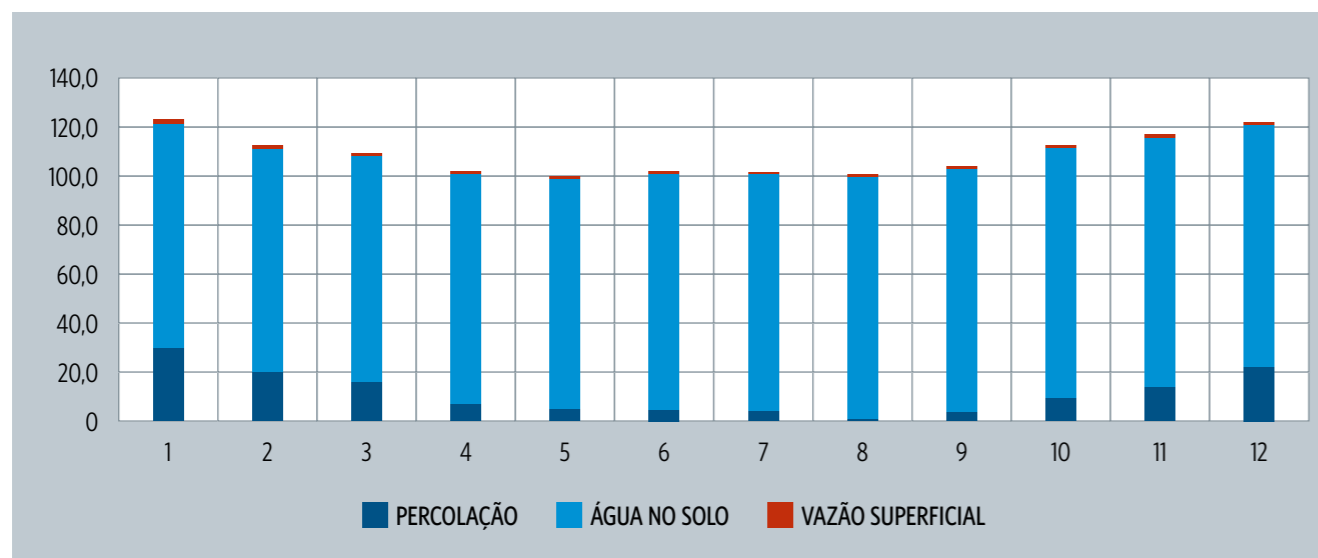
FIGURA 13: DIFERENÇA NA MÉDIA MENSAL DE PERCOLAÇÃO, ÁGUA NO SOLO E ESCOAMENTO SUPERFICIAL ENTRE A LINHA DE BASE E O CENÁRIO RIOS EM MM (2013-2015).
