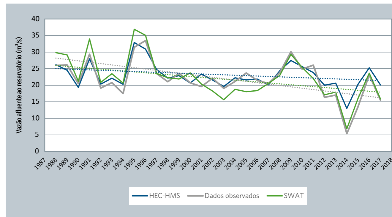
FIGURA 6: COMPARAÇÃO ENTRE AS LINHAS DE BASE DOS MODELOS CALIBRADOS E OS DADOS OBSERVADOS.
