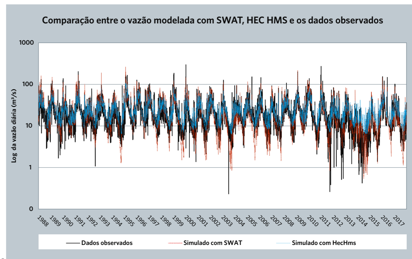
FIGURA 7: PRECISÃO DE RESPOSTA DOS MODELOS SWAT E HEC-HMS EM COMPARAÇÃO COM DADOS OBSERVADOS.
