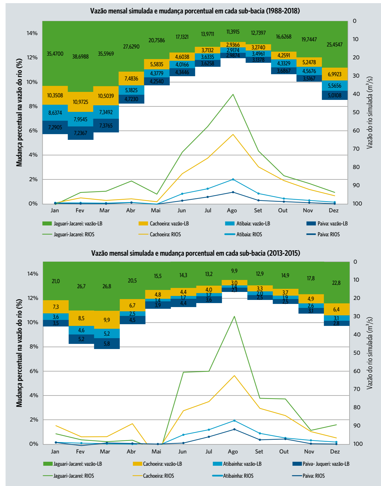
FIGURA 9: VAZÃO MÉDIA MENSAL DO RIO NA LINHA DE BASE (LB) E A ALTERAÇÃO PERCENTUAL DA VAZÃO DEMONSTRADA NO CENÁRIO RIOS NAS SUB-BACIAS. (A) TODO O PERÍODO DE SIMULAÇÃO E (B) ANOS DE SECA
