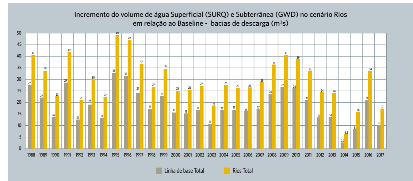
FIGURA 16: INCREMENTO DO VOLUME DE ÁGUA SUPERFICIAL SUBTERRÂNEA NO CENÁRIO RIOS EM RELAÇÃO À LINHA DE BASE CONSIDERANDO AS BACIAS DE DESCARGA
