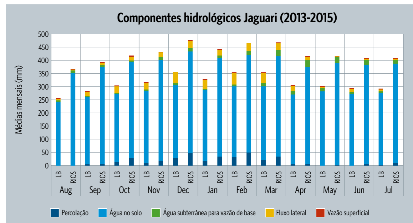
FIGURA 12: MÉDIAS MENSIS DO BALANÇO HÍDRICO SIMULADAS COM O MODELO SWAT PARA O PERÍODO DE SECA DE 2013-2015 (CENÁRIO DE LINHA DE BASE VERSUS CENÁRIO RIOS)
