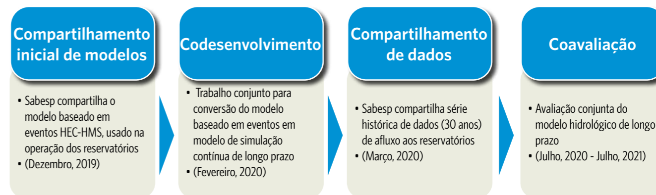
FIGURA 2: PROCESSO DE CODESENVOLVIMENTO DOS MODELOS DE SIMULAÇÃO HIDROLÓGICA DE LONGO PRAZO AO LONGO DO PROJETO, ADAPTANDO A ESTRUTURA DE MODELAGEM HIDROLÓGICA EM USO PELA SABESP
