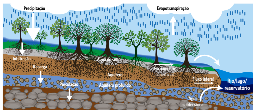
FIGURA 11: PROCESSOS RELACIONADOS À ÁGUA SUBTERRÂNEA NO MODELO SWAT.
