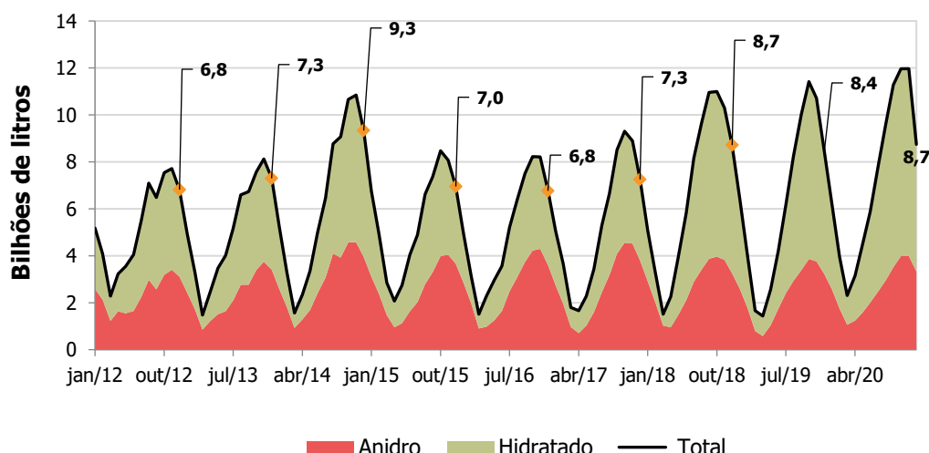
Gráfico 9 - Evolução mensal do estoque físico de etanol
