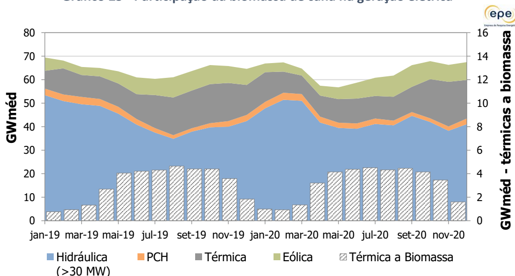
Gráfico 25 - Participação da biomassa de cana na geração elétrica
