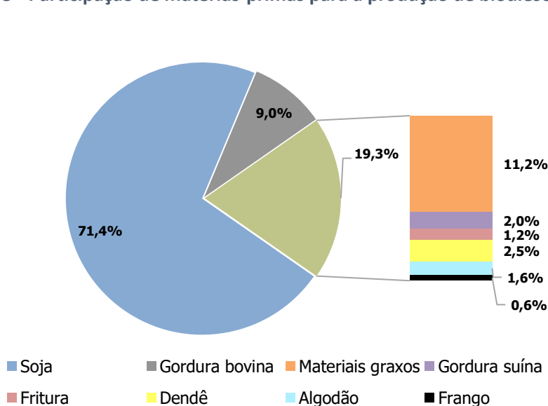
Gráfico 35 - Participação de matérias-primas para a produção de biodiesel em 2020
