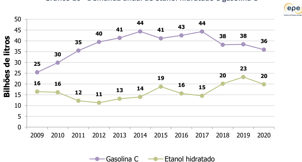
Gráfico 16 - Demanda anual de etanol hidratado e gasolina C
