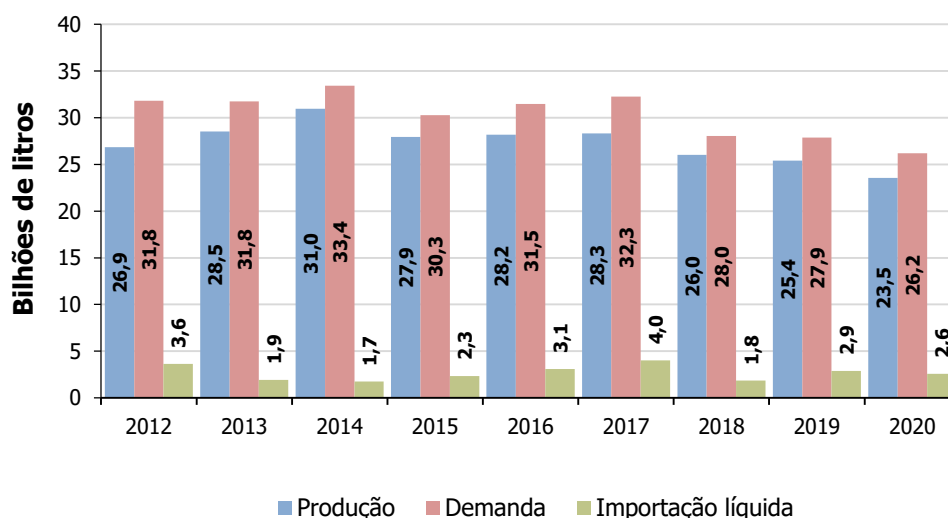
Gráfico 17 - Produção, demanda e importação líquida de gasolina A
