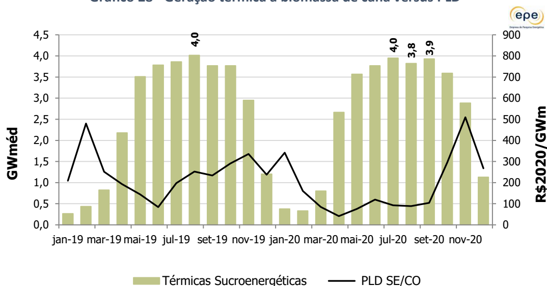
Gráfico 28 - Geração térmica a biomassa de cana versus PLD
