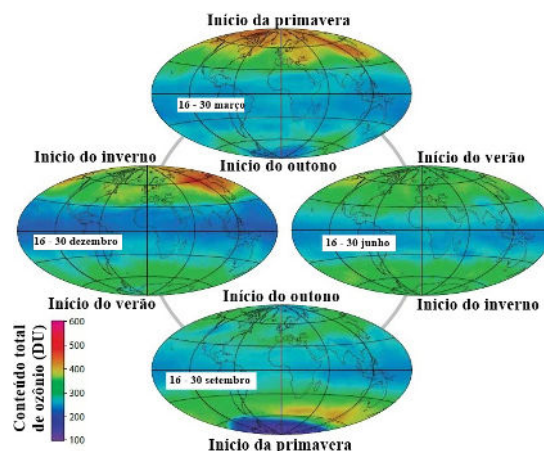
Figura 5. Variabilidade sazonal global do conteúdo total de ozônio (DU). No topo dos painéis é indicada a estação do ano correspondente no hemisfério norte e na base dos painéis, no Hemisfério Sul. Adaptado de Salawitch et al. (2019)
