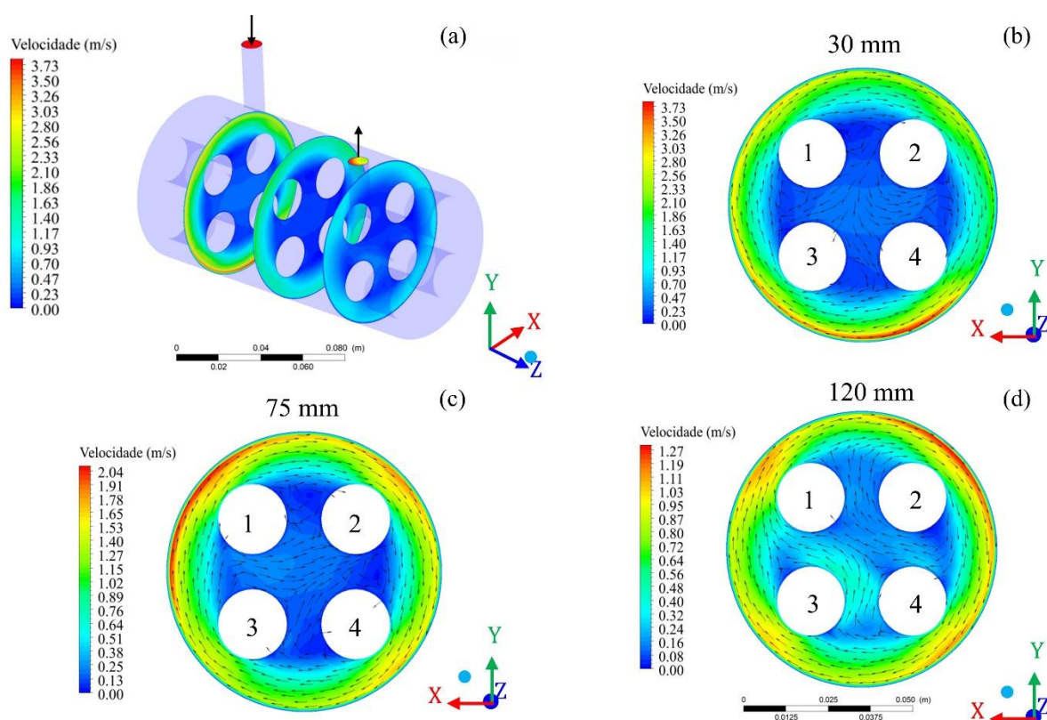
Figura 4.10. Campo de velocidade da mistura em diferentes regiões do casco, (a) vista geral e em z = 30 (b); z = 75 (c) e z = 120 mm (d), do módulo de filtração durante o processo de separação água/óleo (Caso 4).
