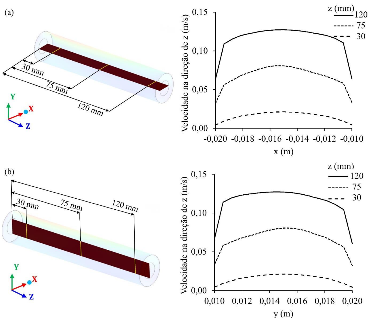
Figura 4.14. Velocidade axial do permeado em diferentes pontos verticais e horizontais ao longo do tubo coletor da membrana, em z = 30, z = 75 e z = 120 mm, do módulo de filtração durante o processo de separação água/óleo (Caso 4).
