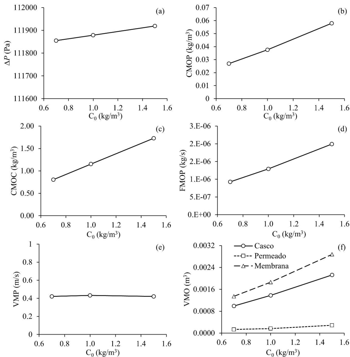
Figura 4.16. Parâmetro do processo no módulo de filtração em função da concentração de óleo na alimentação. (a) Pressão transmembrânica ( \Delta P ), (b) Concentração média de óleo nas saídas dos permeados (CMOP), (c) Concentração média de óleo na saída de concentrado (CMOC), (d) Fluxo médio de óleo nas saídas dos permeados (FMOP), (e) Velocidade média do fluido nas saídas dos permeados (VMP) e (f) Volume médio de óleo (VMO) presente no casco, nas membranas e nos permeados (Casos 5, 6 e 7).
