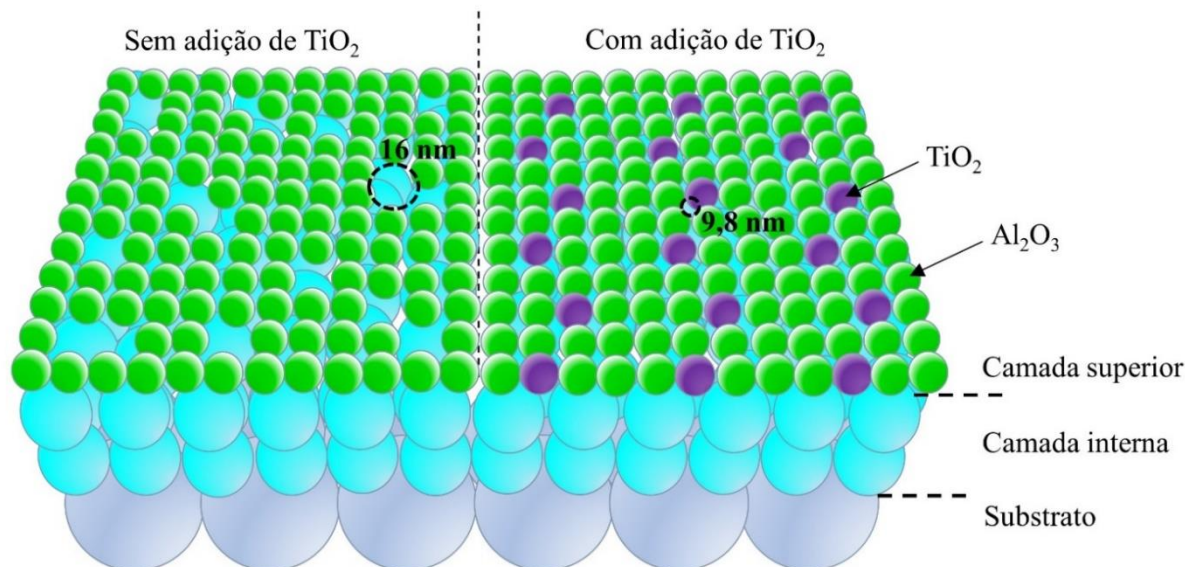
(a) Membrana cerâmica assimétrica típica: processo sol-gel
