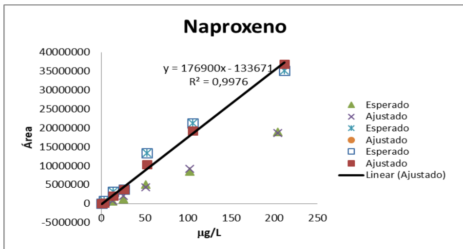
Figura 15- Curva analítica do fármaco naproxeno
