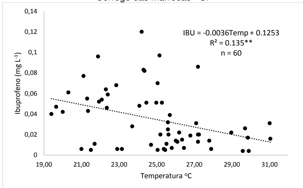
Figura 16- Interação entre ibuprofeno (mg.L -1 ) e temperatura da água (°C) no Córrego das Marrecas - SP
