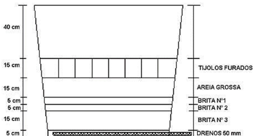
Figura 2. Desenho esquemático do leito de secagem.
