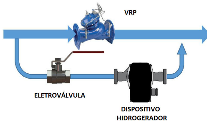
Figura 1: Instalação da microturbina
