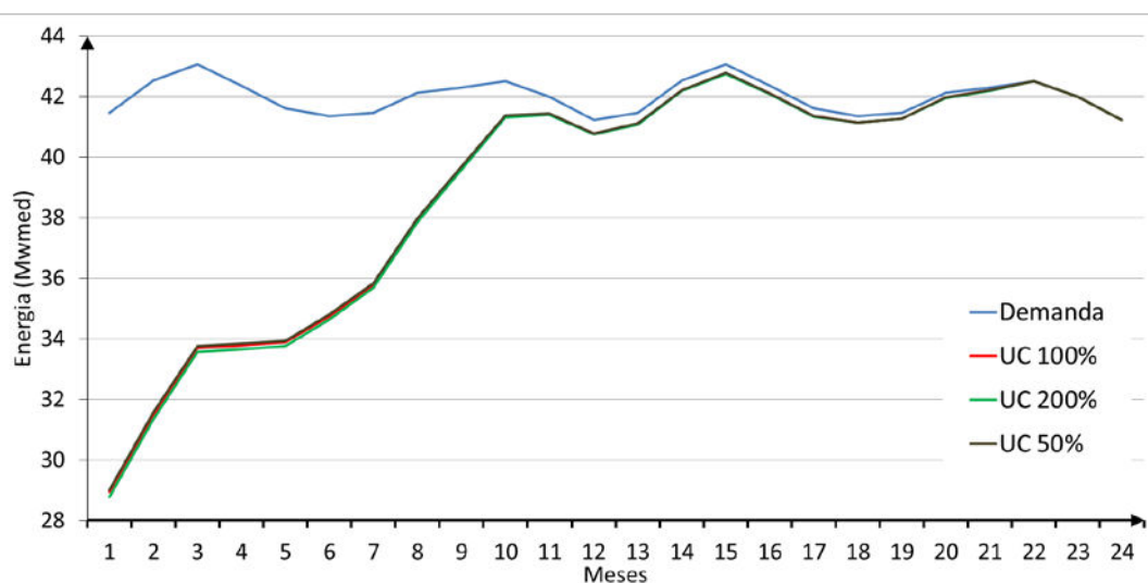
Figura 3: Geração de Energia Elétrica para os Cenários 4, 5 e 6.
