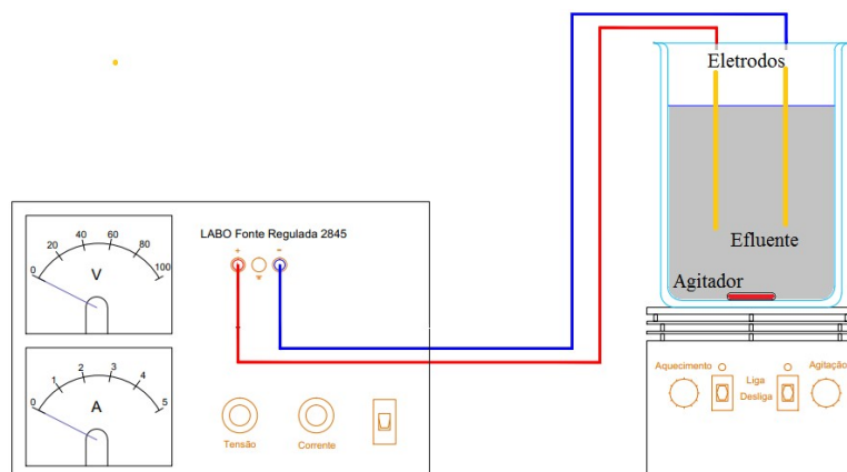
Figura 1 – Reator eletroquímico empregado no experimento.
