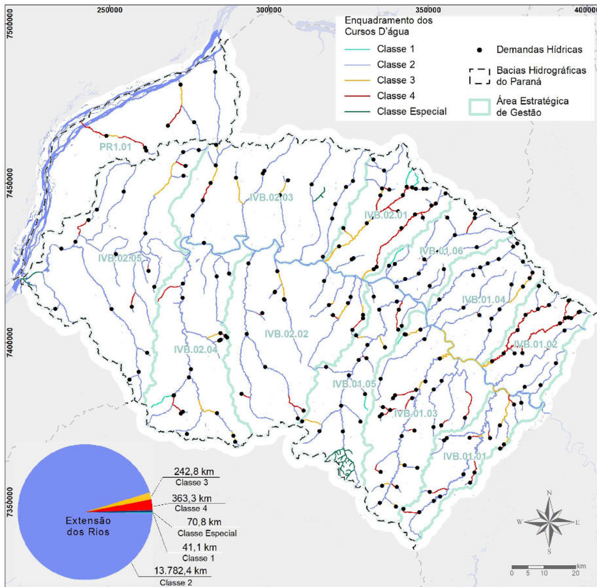
Figura 3: Classes de enquadramento futuro (2025) dos corpos de água por trecho nas bacias hidrográficas do Baixo Ivaí e Paraná 1
