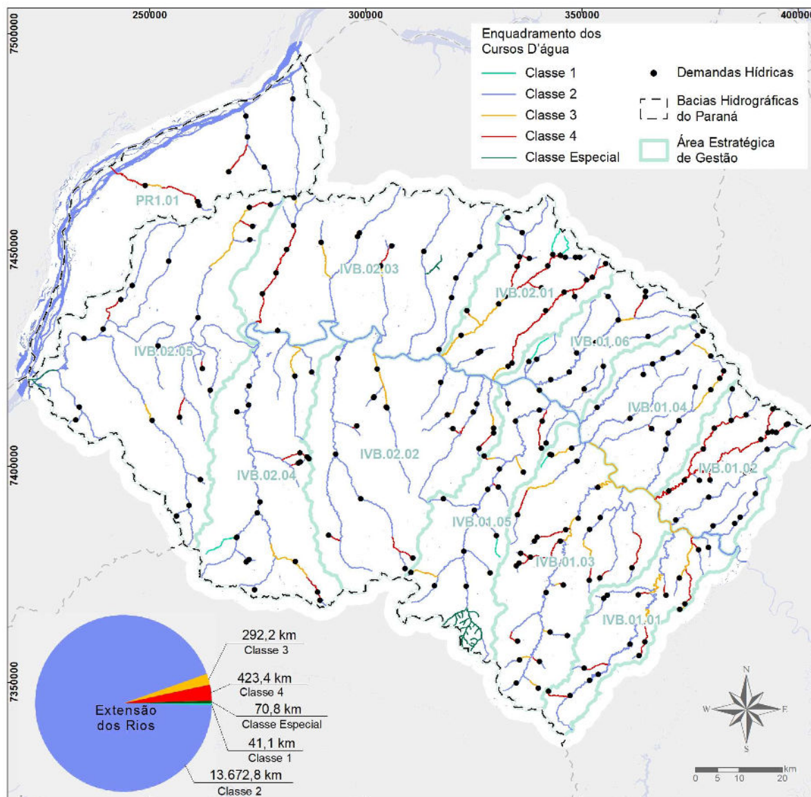
Figura 4: Classes de enquadramento futuro (2030) dos corpos de água por trecho nas bacias hidrográficas do Baixo Ivaí e Paraná 1
