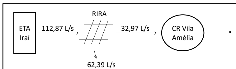
Figura 3: Situação de consumo no sistema após aplicação da Ação 1 com Objetivo 1
