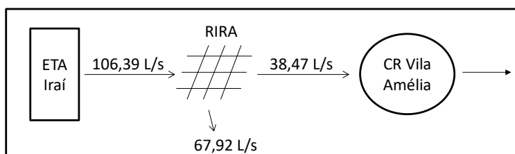
Figura 6: Situação de consumo após aplicação da Ação 2 com Objetivo 2
