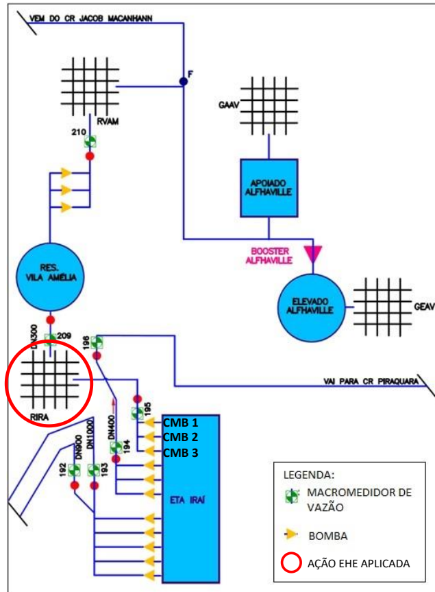
Figura 1: Croqui esquemático do Sistema Iraí – Vila Amélia – Alphaville. Fonte: SANEPAR, 2014.
