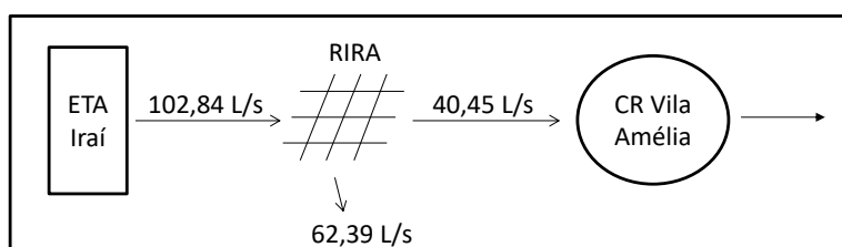
Figura 4: Situação de consumo no sistema após aplicação da Ação 1 com Objetivo 2
