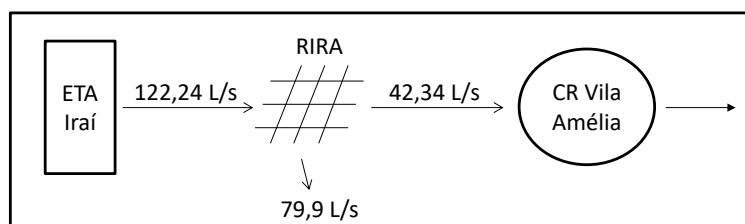
Figura 8: Situação de consumo após aplicação da Ação 3 com Objetivo 2
