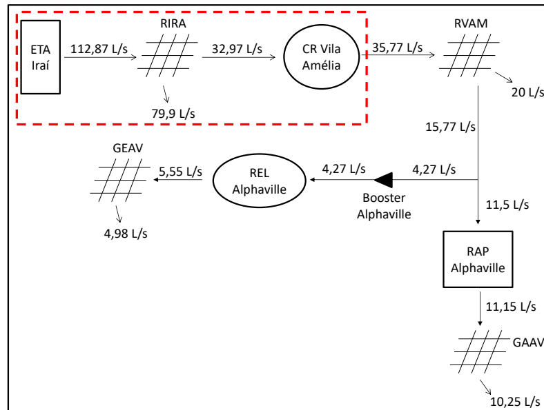
Figura 2: Situação de consumo do Sistema Iraí – Vila Amélia – Alphaville no dia de maior consumo (13/12/2016).
