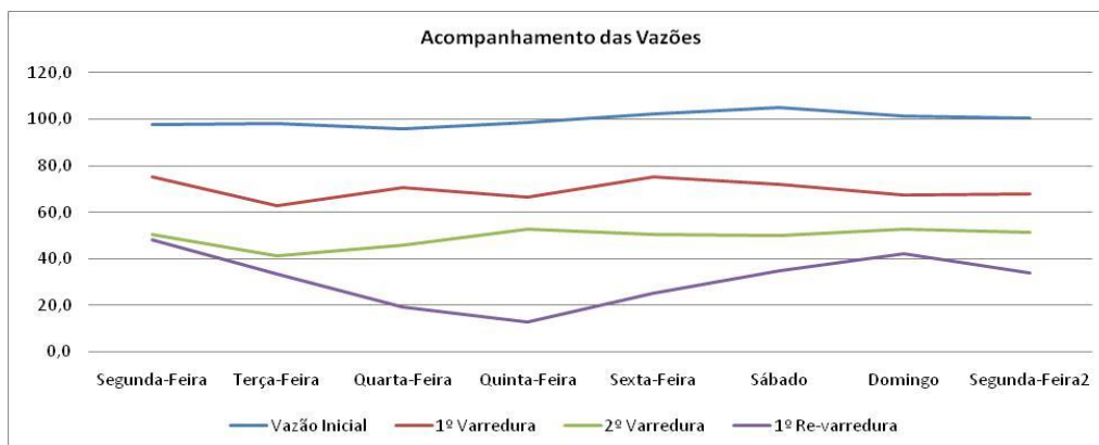
Figura 05 – Diminuição da Vazão Mínima Noturna por Varredura Realizada
