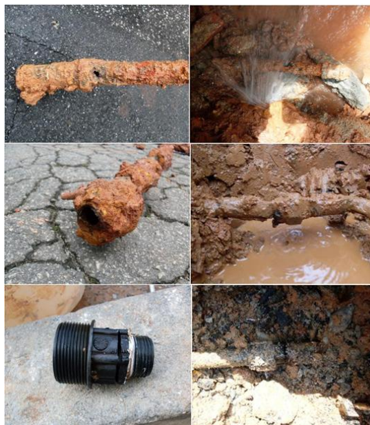
Figura 03– Problemas de infraestrutura encontrados
