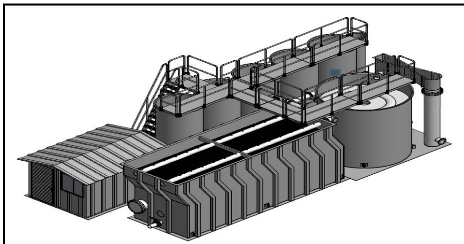
Figura 1: Vista isométrica da Estação de Tratamento de Água Bom Conselho
