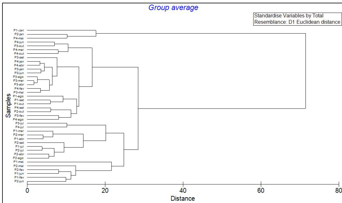
Figura 2. Análise de Agrupamentos Hierárquicos nos dados físicos, químicos e microbiológicos nas Lagoas do Norte em dez períodos de avaliação (de janeiro a outubro de 2016). O dendograma foi construído pela distância euclidiana
