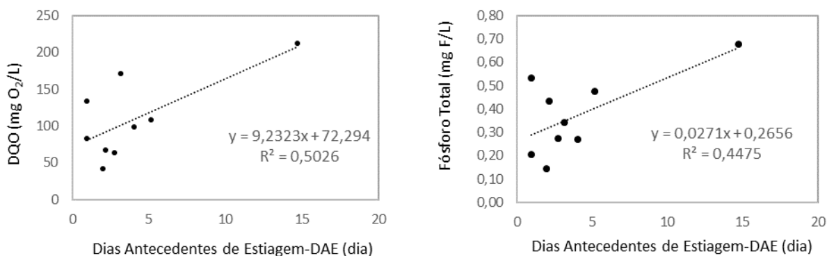
Figura 2: Regressão linear simples entre Dias Antecedentes de Estiagem, DQO e Fósforo Total.
