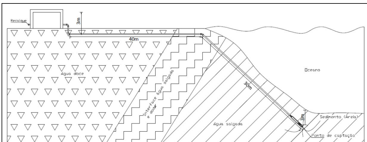
Figura 3: Perfil construtivo sistema de captação angular de água salina.
