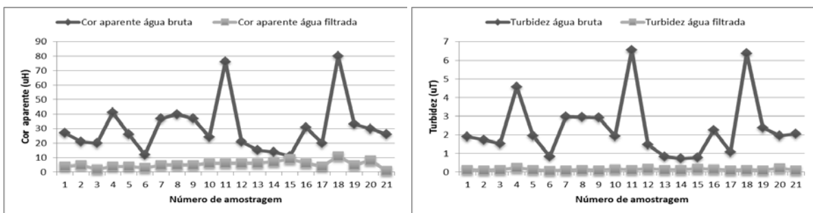
Figura 5: Turbidez e Cor aparente da água bruta e água filtrada pelo sistema angular.
