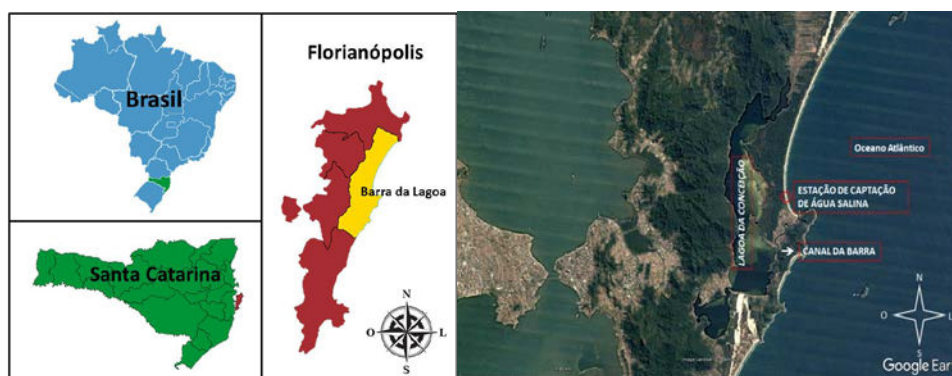
Figura 1: Localização da estação de captação salina, Barra da Lagoa, Florianópolis/SC.
