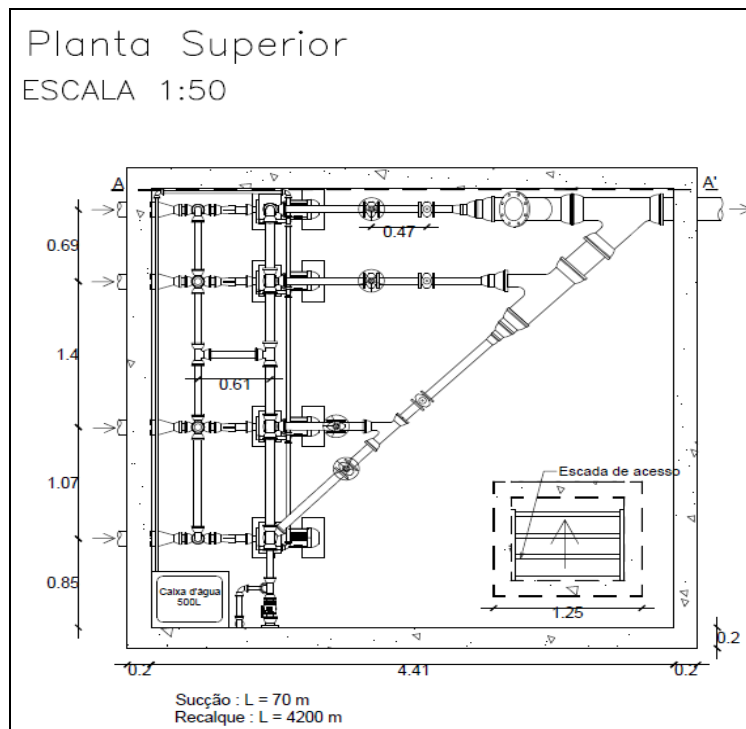
Figura 2: Planta superior do sistema de captação angular de água salina.
