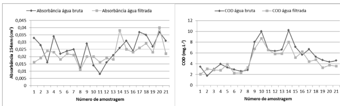
Figura 6: Absorbância 254nm e COD da água bruta e água filtrada pelo sistema angular
