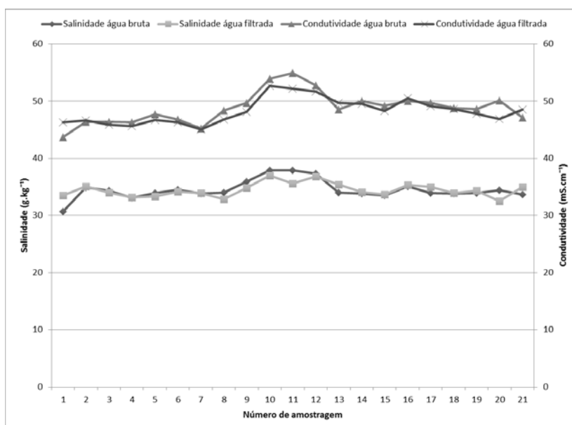
Figura 4: Salinidade e Condutividade da água bruta e água filtrada pelo sistema angular.
