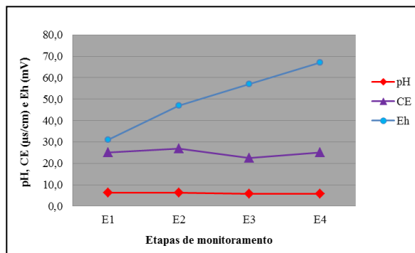
Figura 8 – Gráfico de pH, CE e Eh para o ponto IU-02, representante da Bacia do Igarapé Aracu, na primeira (E1), segunda (E2), terceira (E3) e quarta etapa (E4) de monitoramento.
