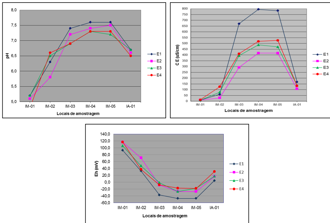
Figura 5 – Gráficos com valores de pH, condutividade elétrica (CE) e potencial de oxi-redução (Eh), medidos em campo, nas amostras coletadas na Bacia Matrinxã-Acará na primeira (E1), segunda (E2), terceira (E3) e quarta etapas (E4) desta terceira fase de monitoramento.
