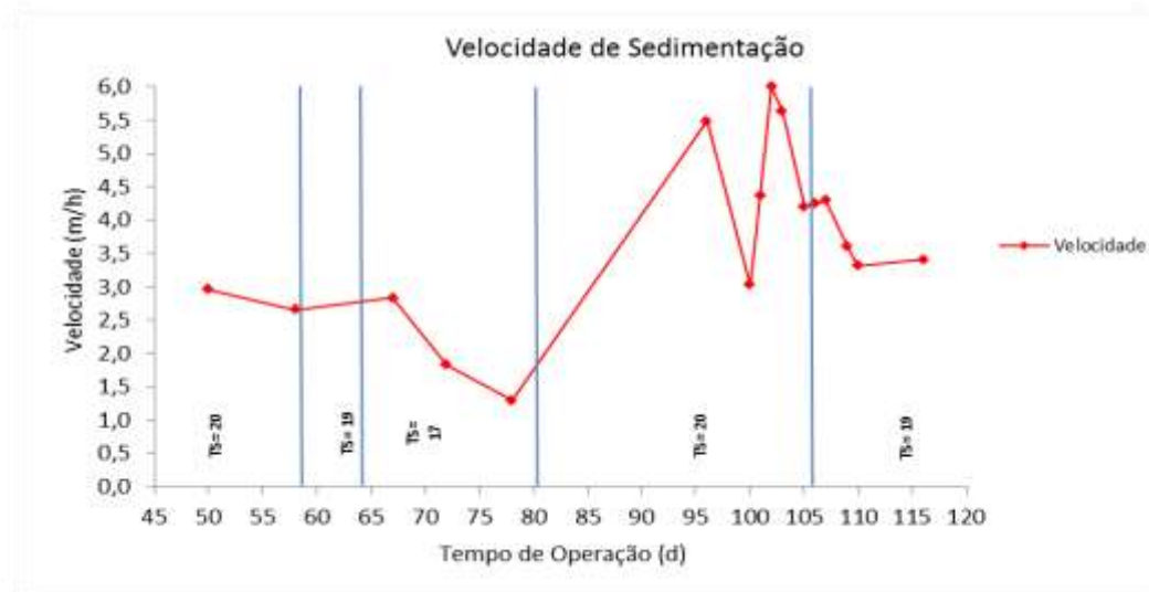
Figura 9: Velocidade de sedimentação dos flocos aeróbios.
