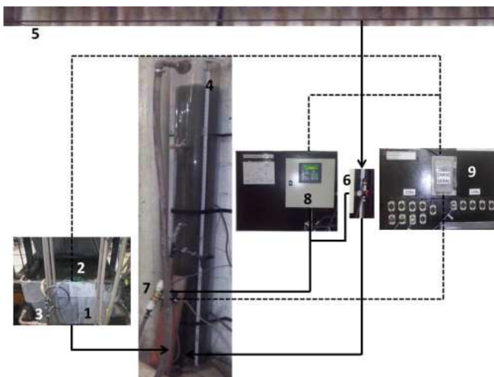
Figura 1: Sistema Experimental.
