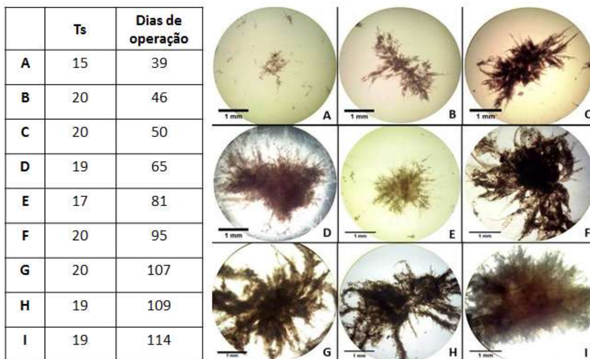
Figura 7: Desenvolvimento dos Grânulos Aeróbios.
