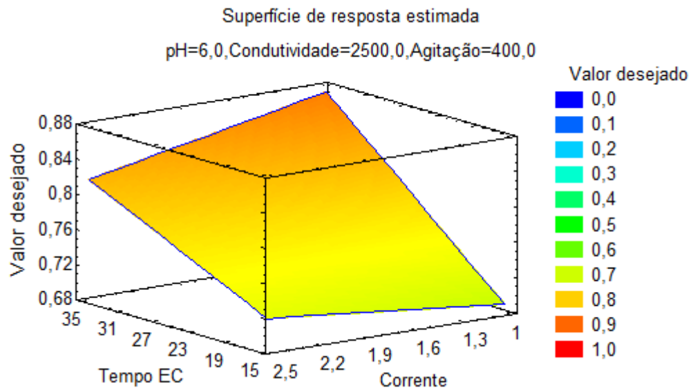
Figura 27 - Superfície de resposta para a remoção do fósforo em função do tempo e da corrente.
