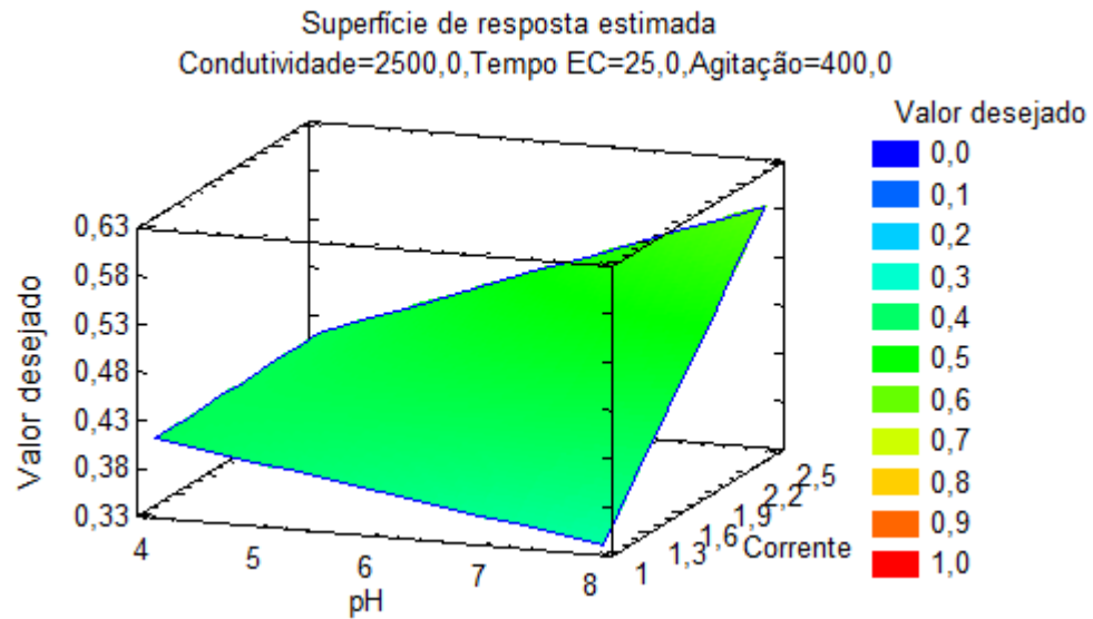
Figura 30 - Superfície de resposta para a remoção de nitrato em função do pH e da corrente.
