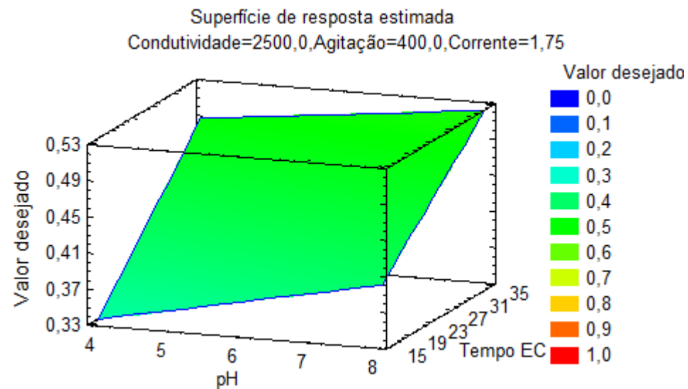
Figura 31 - Superfície de resposta para a remoção de nitrato em função do pH e do tempo.
