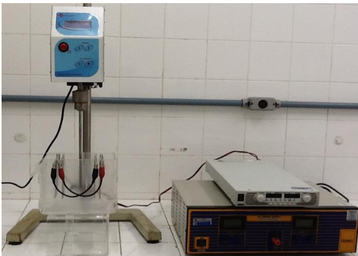
Figura 14 - Desenho da linha experimental de eletrocoagulação.
