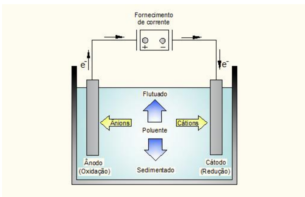
Figura 9 - Reator eletroquímico.
