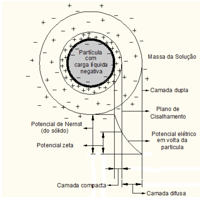
Figura 2 – Dupla camada e potenciais elétricos desenvolvidos ao redor da partícula.
